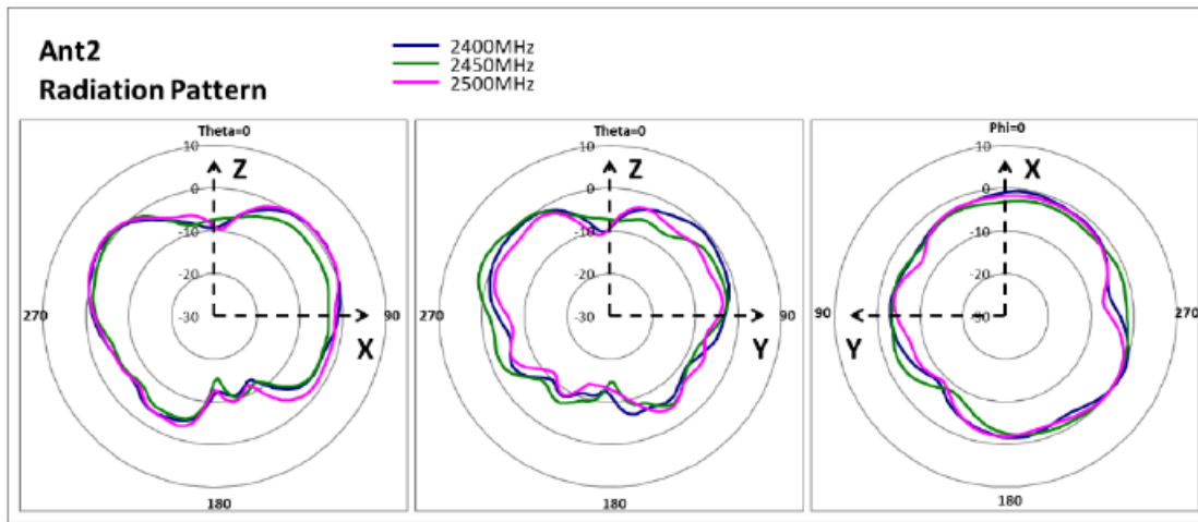
ANTENNA 2 (2GHz)
