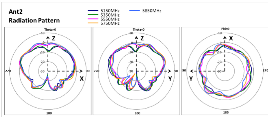
ANTENNA 2 (5GHz)
