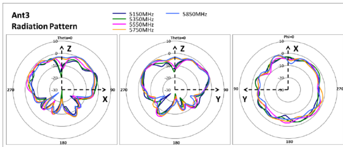
ANTENNA 3 (5GHz)
