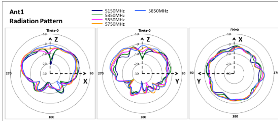
ANTENNA 1 (5GHz)
