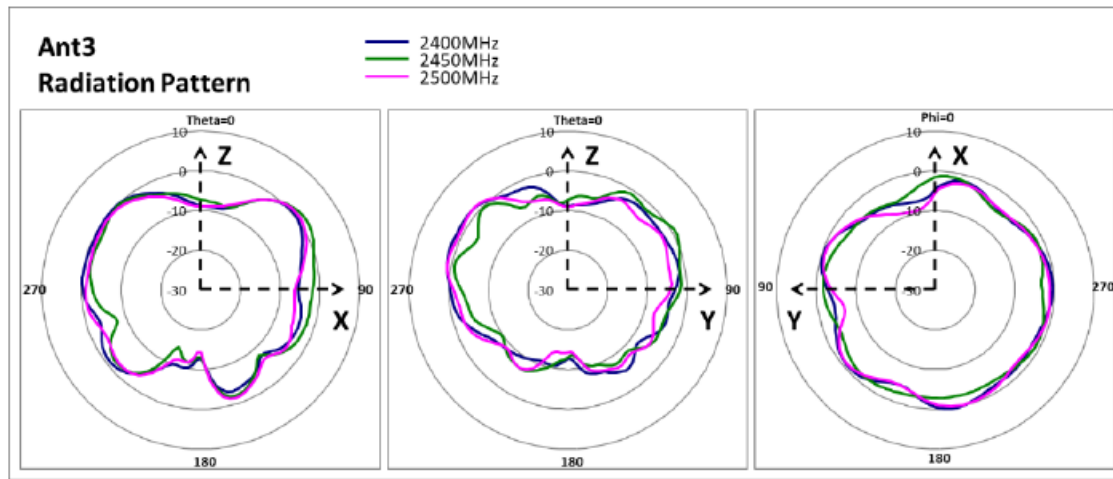
ANTENNA 3 (2GHz)
