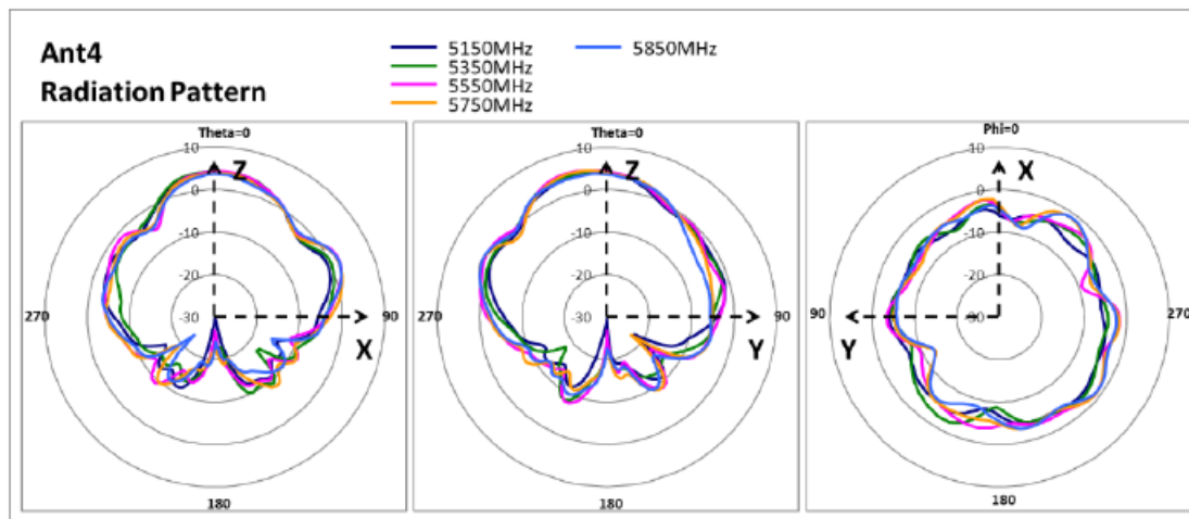
ANTENNA 4 (5GHz)
