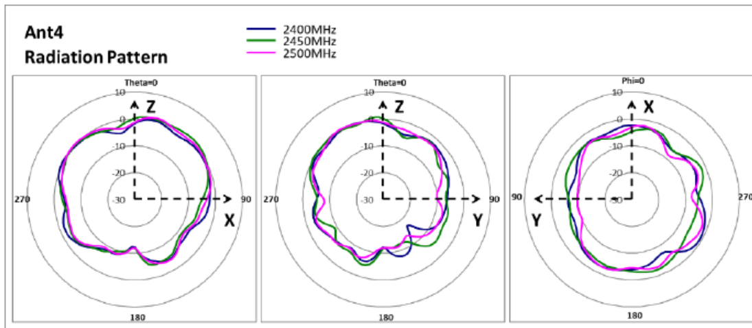
ANTENNA 4 (2GHz)
