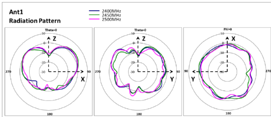
ANTENNA 1 (2GHz)
