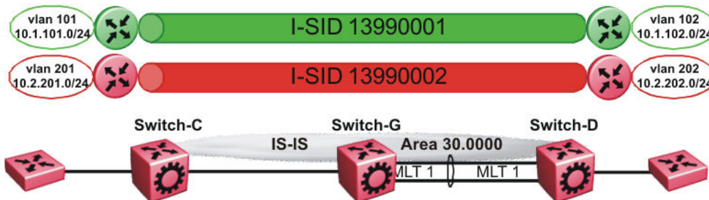
Figure 56: Layer 3 VSN
