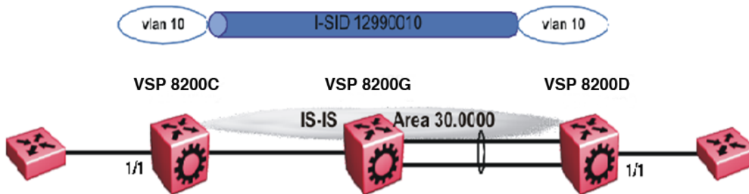
Figure 46: Layer 2 VSN
