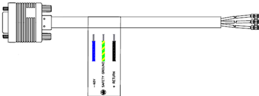
Рисунок 3: Кабель питания пост. тока
