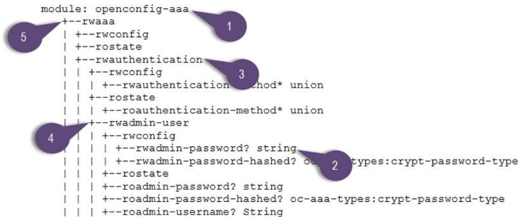
Figure 2: YANG Data Model Components
