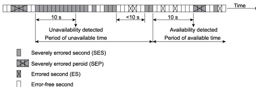
Figure 163: SES
