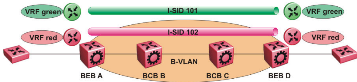
Figure 133: SPBM Layer 3 VSN
