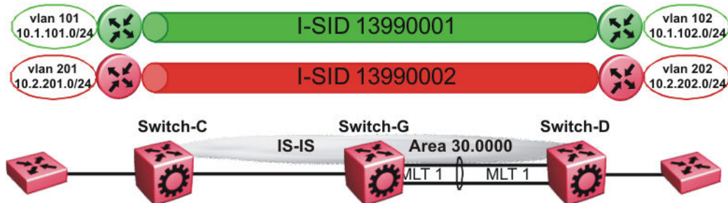
Figure 135: Layer 3 VSN
