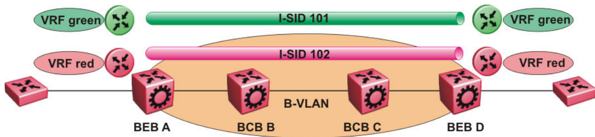
Figure 122: SPBM Layer 3 VSN
