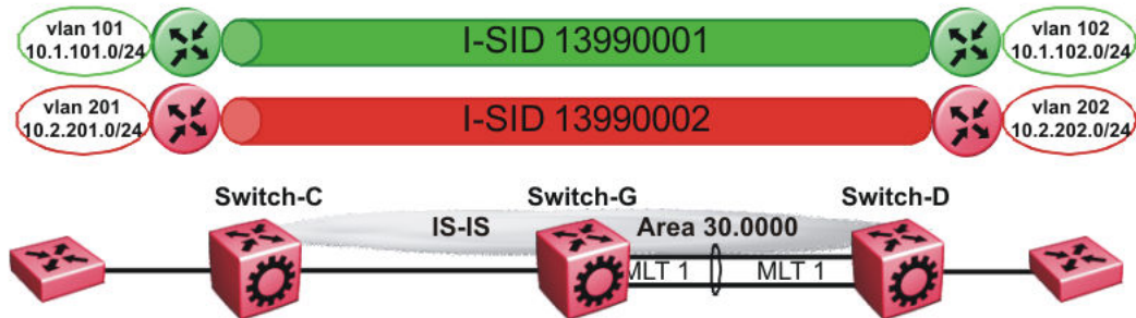
Figure 119: Layer 3 VSN
