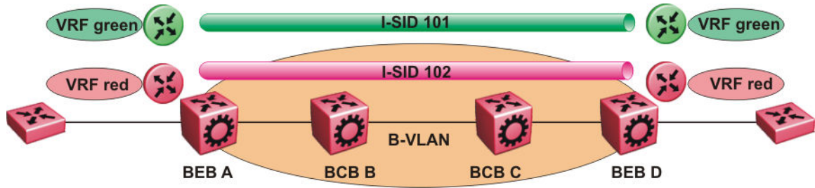
Figure 117: SPBM Layer 3 VSN
