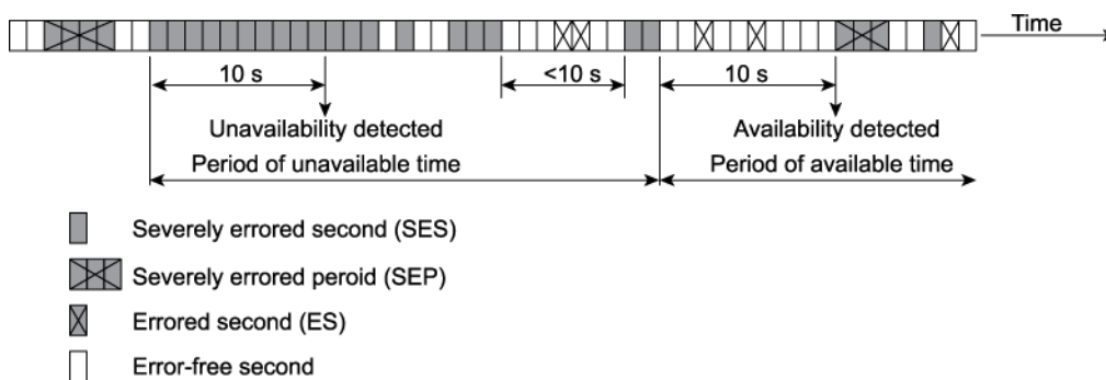
Figure 54: SES
