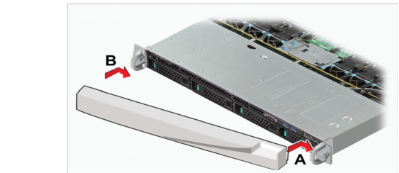
图 4 安装可选挡板
