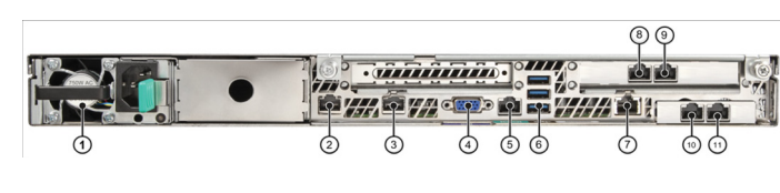
图 1 E2120 后面板布局
