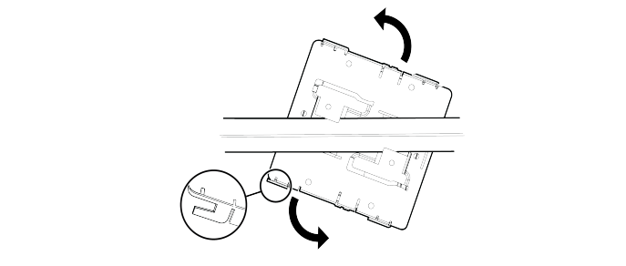
Figura 2 Fijación del soporte de montaje principal a un perfil en T
